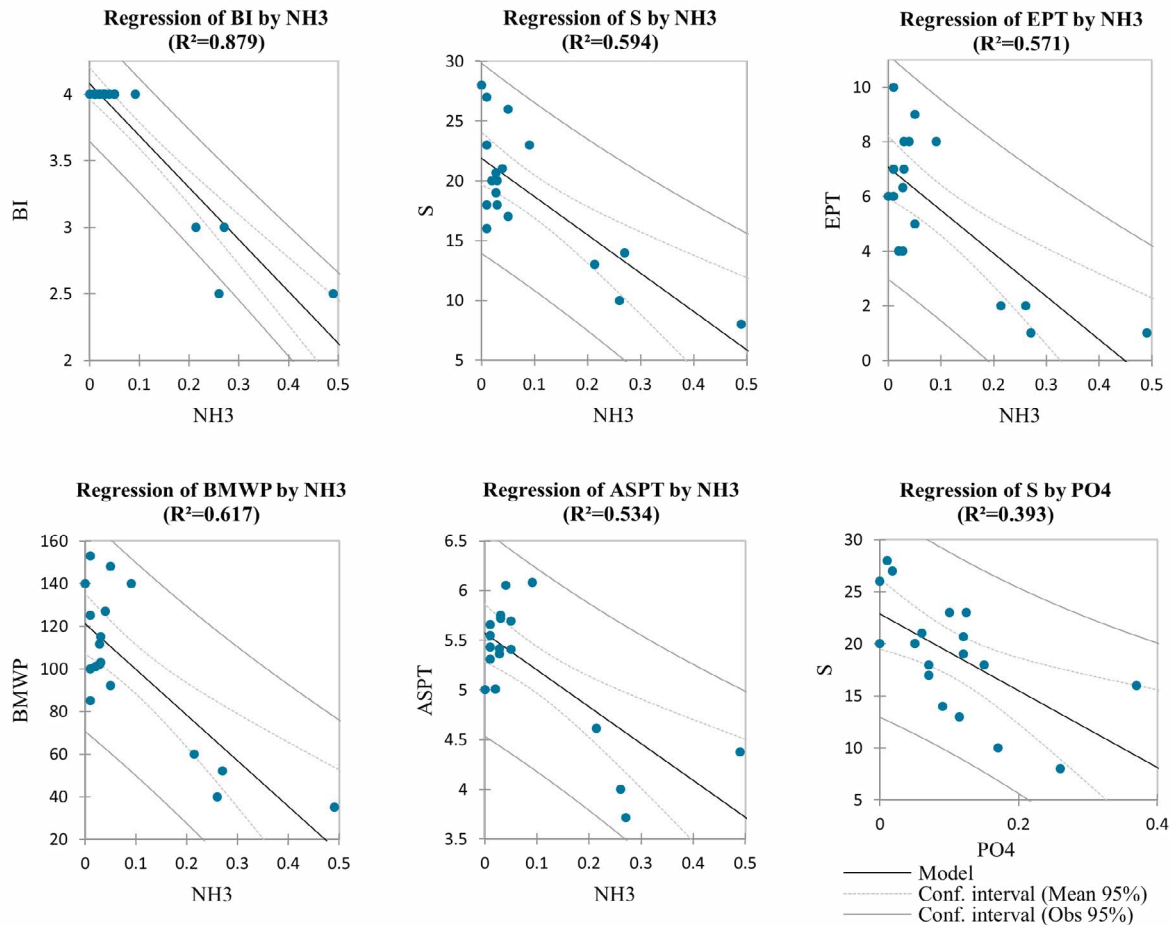
Figure 9. Linear regression analysis between physicochemical parameters from the river and biomonitoring metrics. Análisis de regresión lineal entre parámetros físicoquímicos del río y métricas de biomonitoreo.
