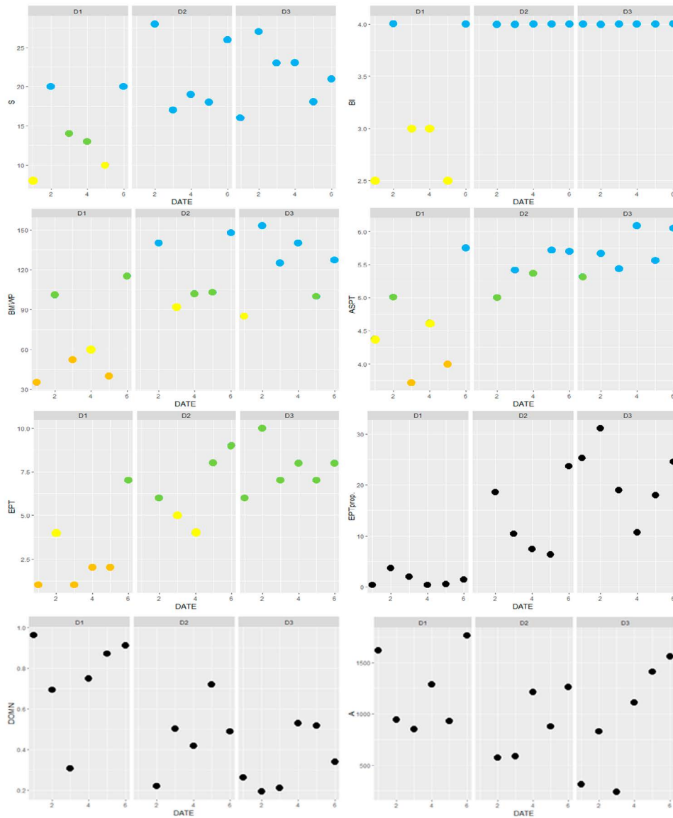
Figure 8. Temporal and spatial dynamics of the biological indices: BMWP, ASPT, EPT, EPTprop. - Ratio between the abundance of EPT individuals and total invertebrate abundance, BI, S, DOMN, and A. Color coding of the ecological status assessment in the figure: blue – high ecological status; green – good ecological status; yellow – moderate ecological status; orange – poor ecological status. Dinámica espacial y temporal de los índices biológicos: BMWP, ASPT, EPT, EPTprop. - Ratio entre la abundancia de individuos del EPT y la abundancia total de invertebrados, BI, S, DOMN y A. Codificación de colores de la evaluación del estado ecológico en la figura: azul – buen estado ecológico; verde – buen estado ecológico; amarillo – estado ecológico moderado; naranja – deficiente estado ecológico.
